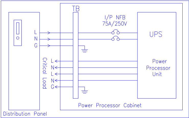
Fig a.C-8000,C-10000,C-12000 機配線圖.
