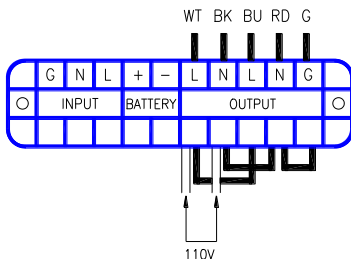
Fig e. 1Ø 2W 110V
