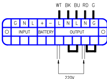
Fig d. 1Ø 2W 220V
