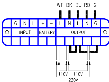
Fig f. 1Ø 3W
