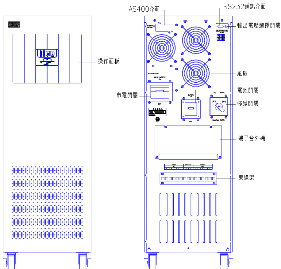
3C-10000,3C-12000外觀圖
