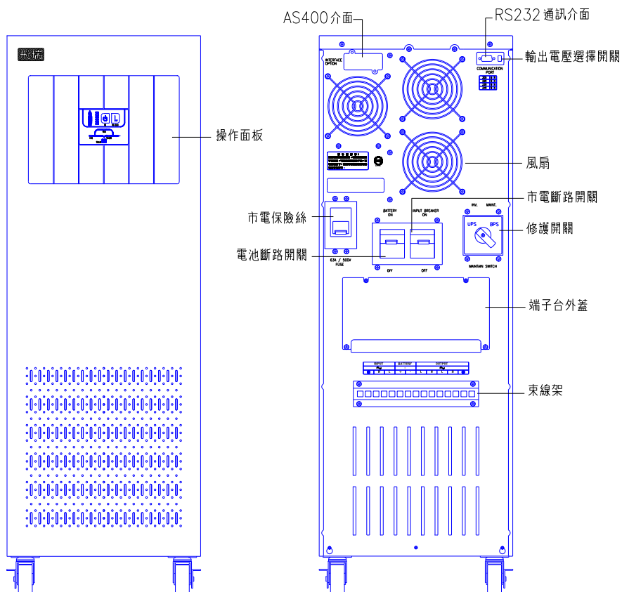
C-8000,C-10000,C-12000外觀圖
