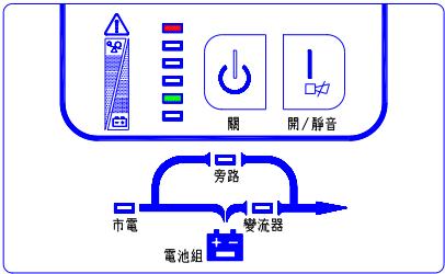
(電池供電狀態)
